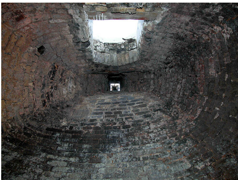
En af de kubeformede kalkovne set indefra og op gennem skorstenen mod indfyldningshullet.
